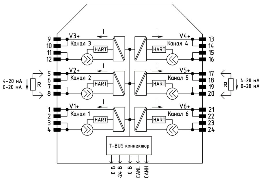
Рисунок 46 – Схема подключения модуля K15.AO6.HART
