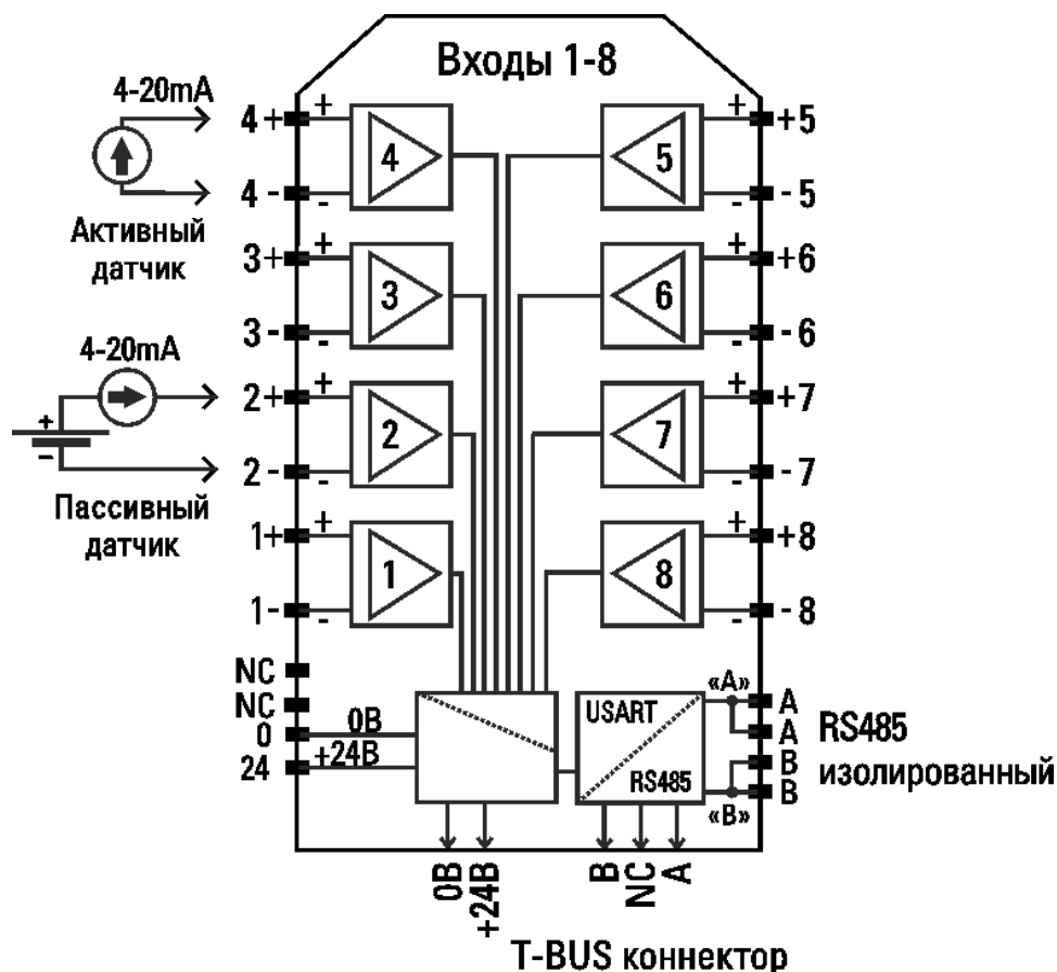
Рисунок 34 - Схема подключения модуля K15.AI8.RS
