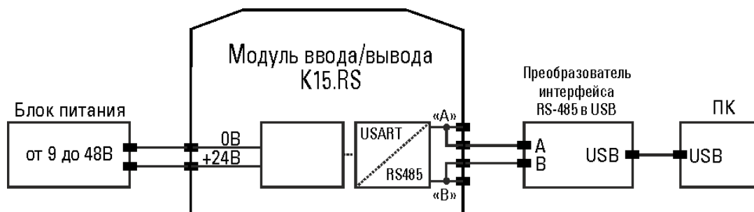
Рисунок 54 – Подключение модуля к ПК
