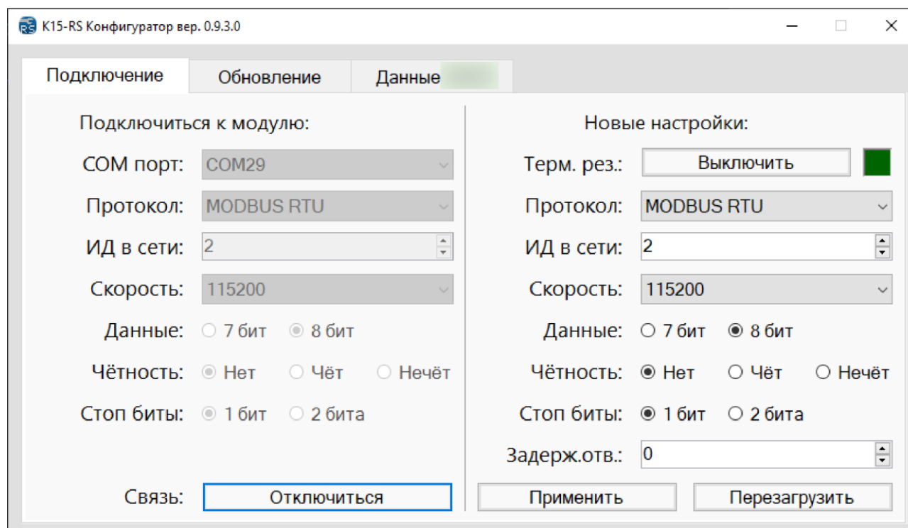
Рисунок 56 – Подключение модулей RS
