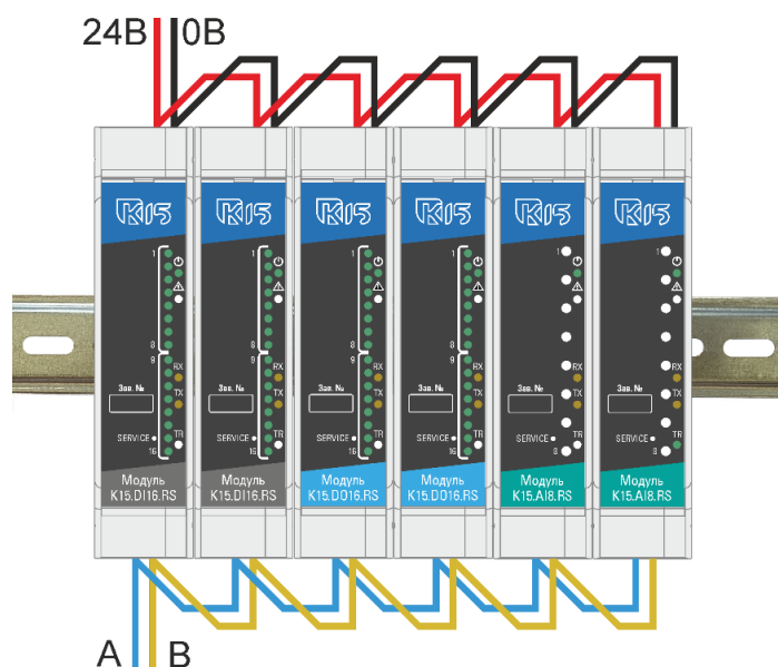
Рисунок 53 – Схема подключения шин питания и связи при подключении группы модулей без шинных соединителей T-BUS
