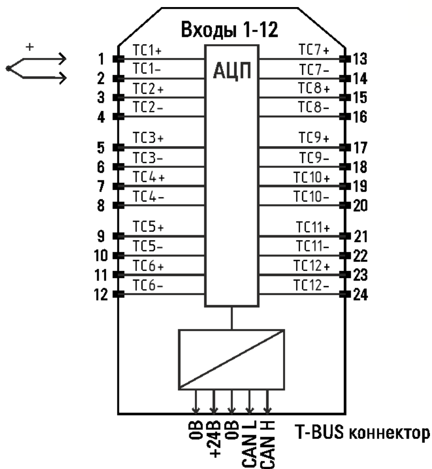
Рисунок 39 - Схема подключения модуля K15.TC12
