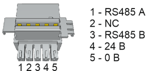
Рисунок 51 – Шинный соединитель T-BUS для модулей с интерфейсом связи RS
