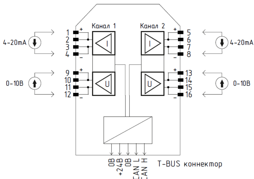
Рисунок 43 – Схема подключения модуля К15.АО2
