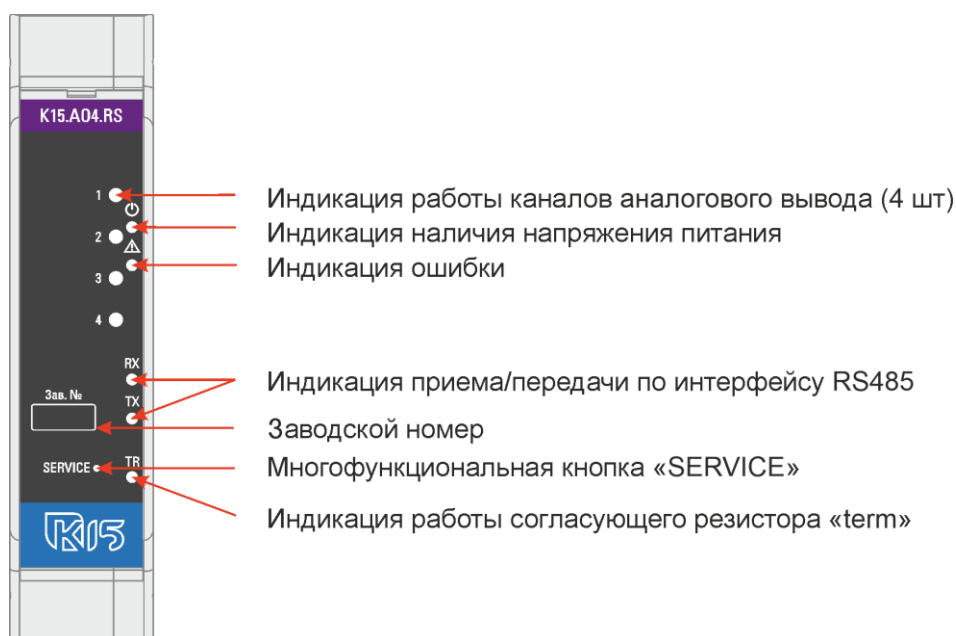
Рисунок 42 – Передняя панель модуля K15.AO4.RS
