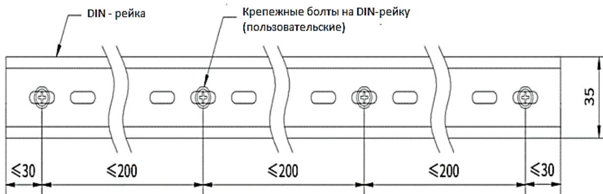
Рисунок 48 – Расположение крепежных болтов
