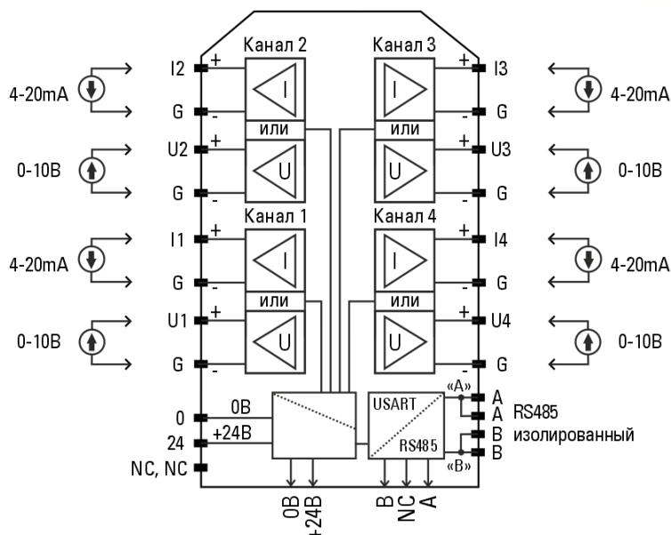
Рисунок 45 – Схема подключения модуля
