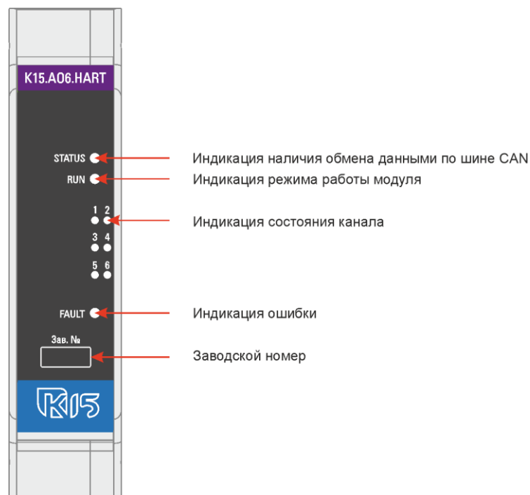
Рисунок 41 – Передняя панель модуля K15.AO6.HART
