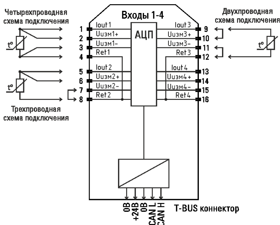
Рисунок 38 - Схема подключения модуля K15.TR4
