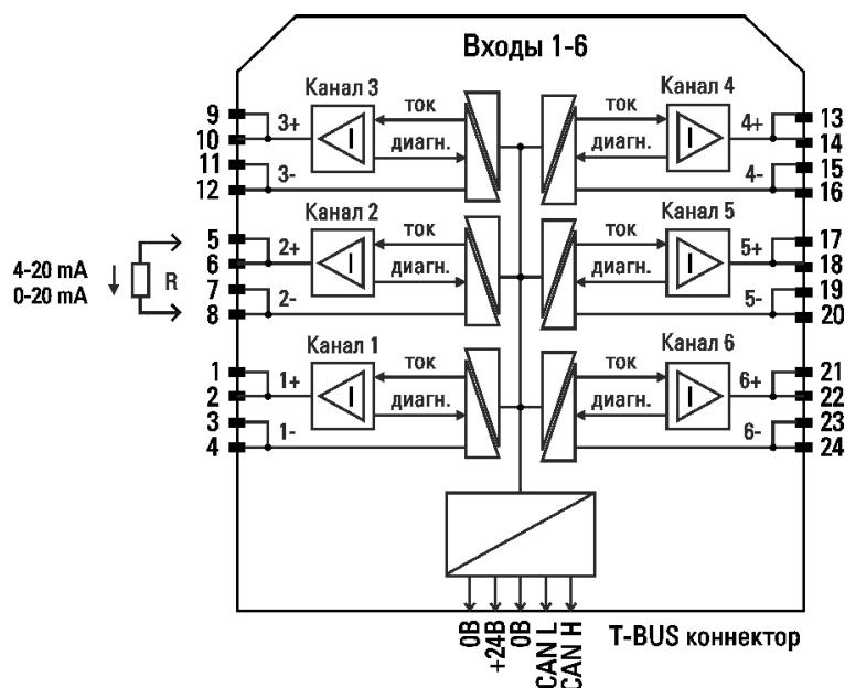
Рисунок 44 – Схема подключения модуля K15.AO6
